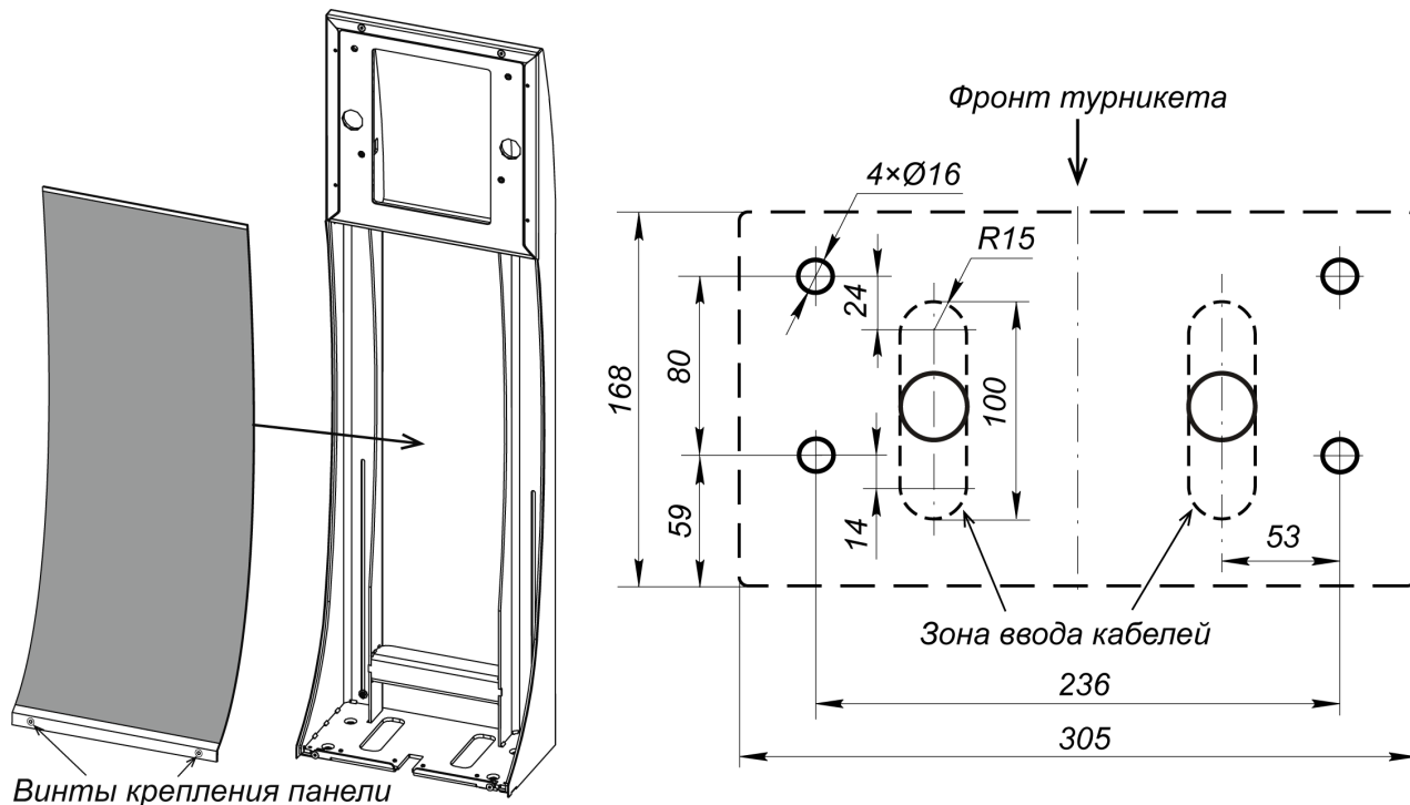
Рисунок 19. Порядок монтажа и схема разметки отверстий для стойки PERCo-MT10.3 1
