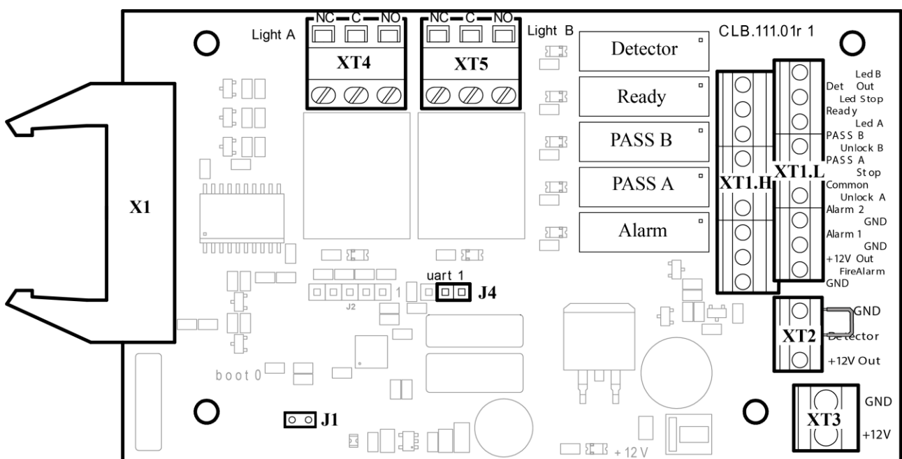
Рисунок 5. Внешний вид платы управления CLB
