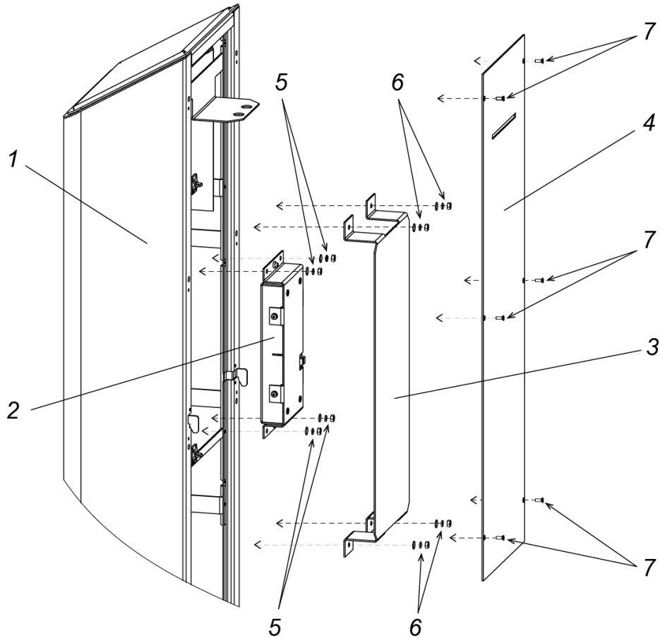
Рисунок 20. Блок постоянной индикации стандартного бокового модуля
