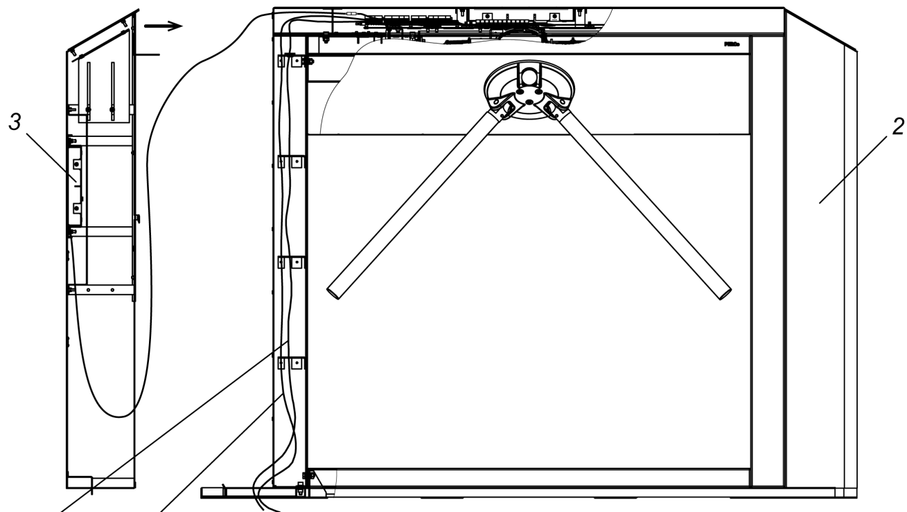
Вид сверху со снятой крышкой
