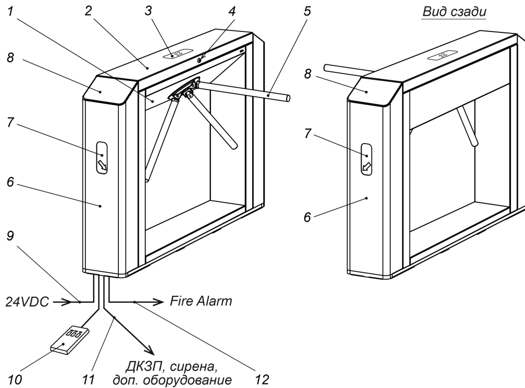
Стандартная модификация PERCo-TTD-12AB
