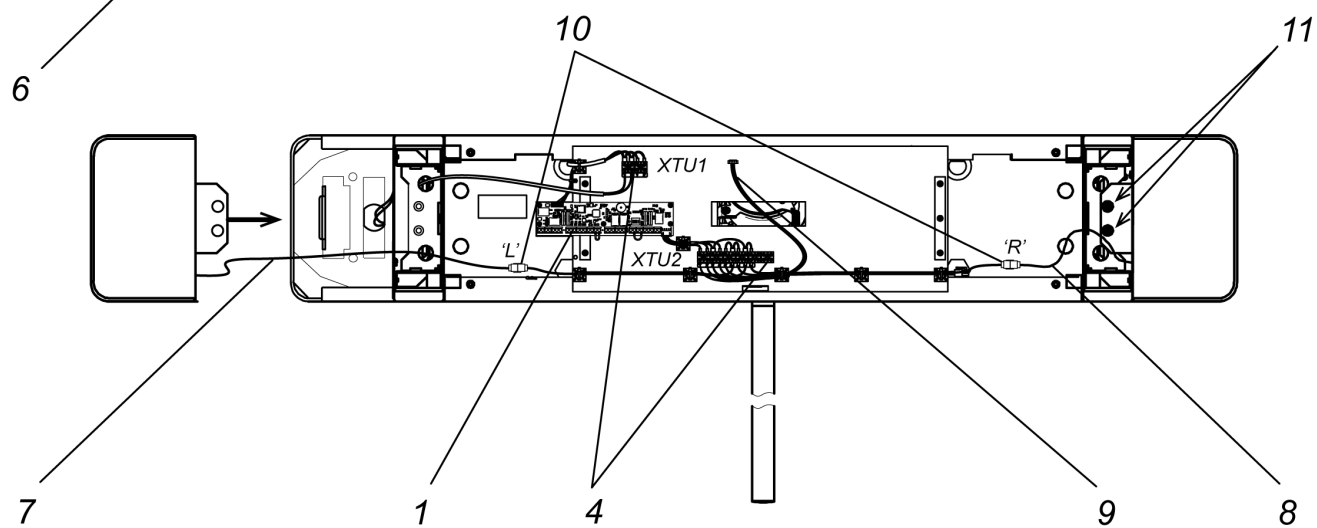
Рисунок 19. Схема прокладки кабелей в стойке турникета
