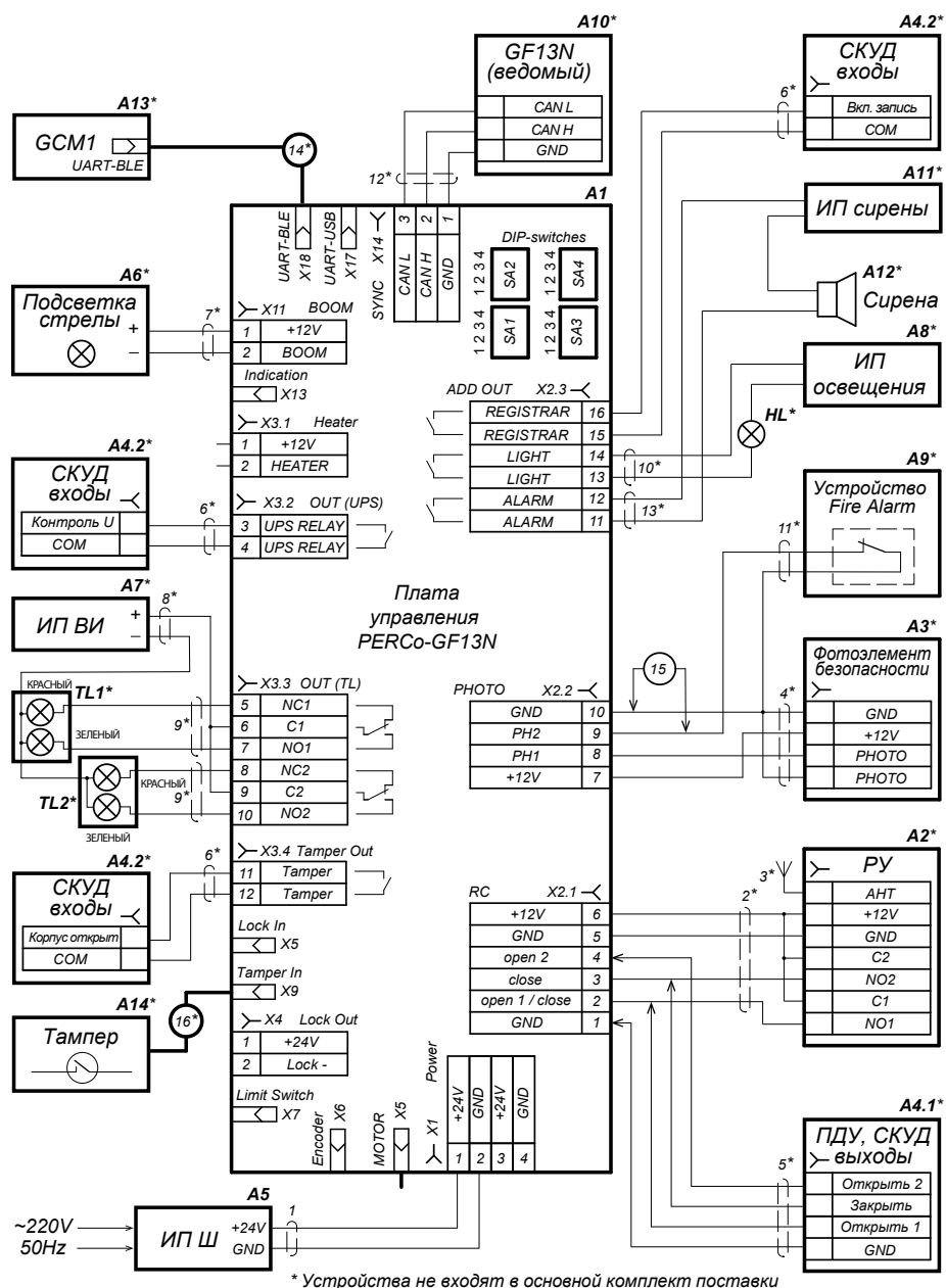
Схема электрических соединений шлагбаума GF13N
