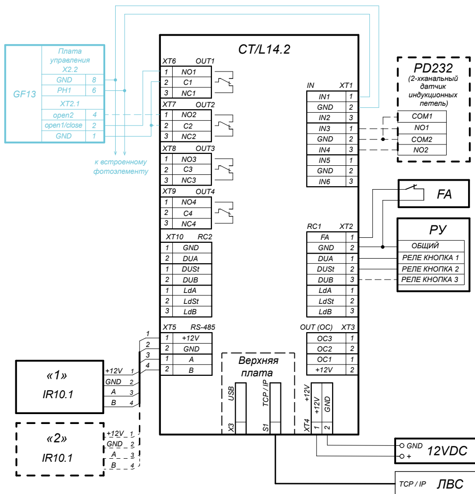
Пунктиром показан вариант реализации двухстороннего управления проездом Пример схемы подключения к контроллеру СКУД
